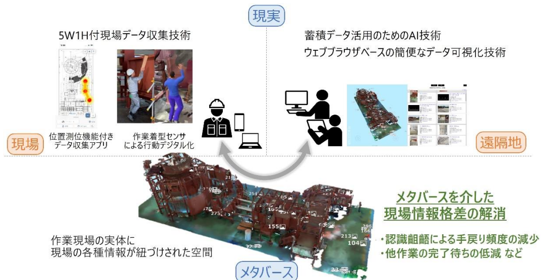
実際の工事における現場拡張メタバースの適用イメージ
